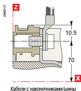
CVS100 - 250
