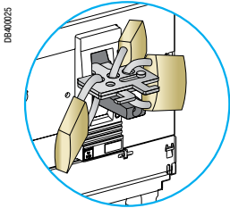
Блокировка рычага управления с помощью специального устройства и навесных замков: Съемное устройство
