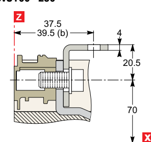
CVS100 - 250
