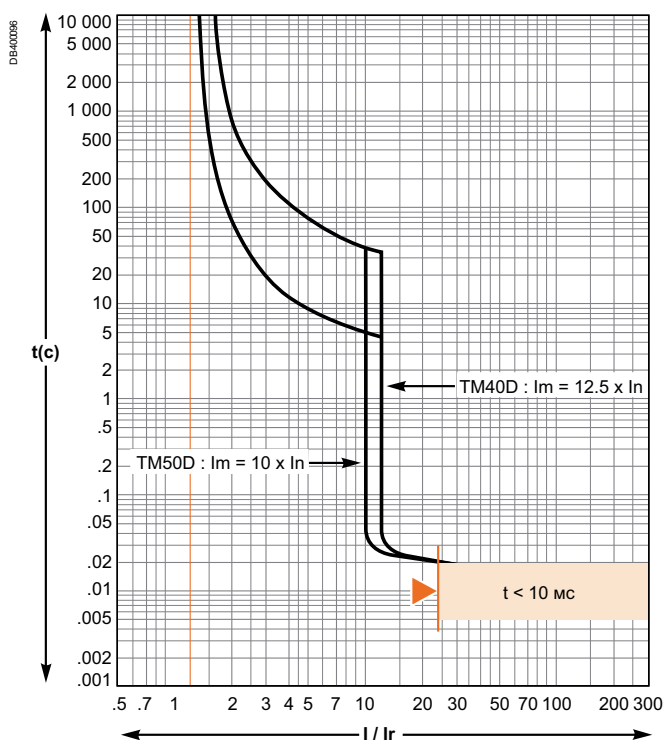
TM40D/50D
