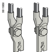
Детали монтажа: 2 кабеля с наконечниками
