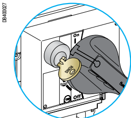
Блокировка поворотной рукоятки встроенным замком
